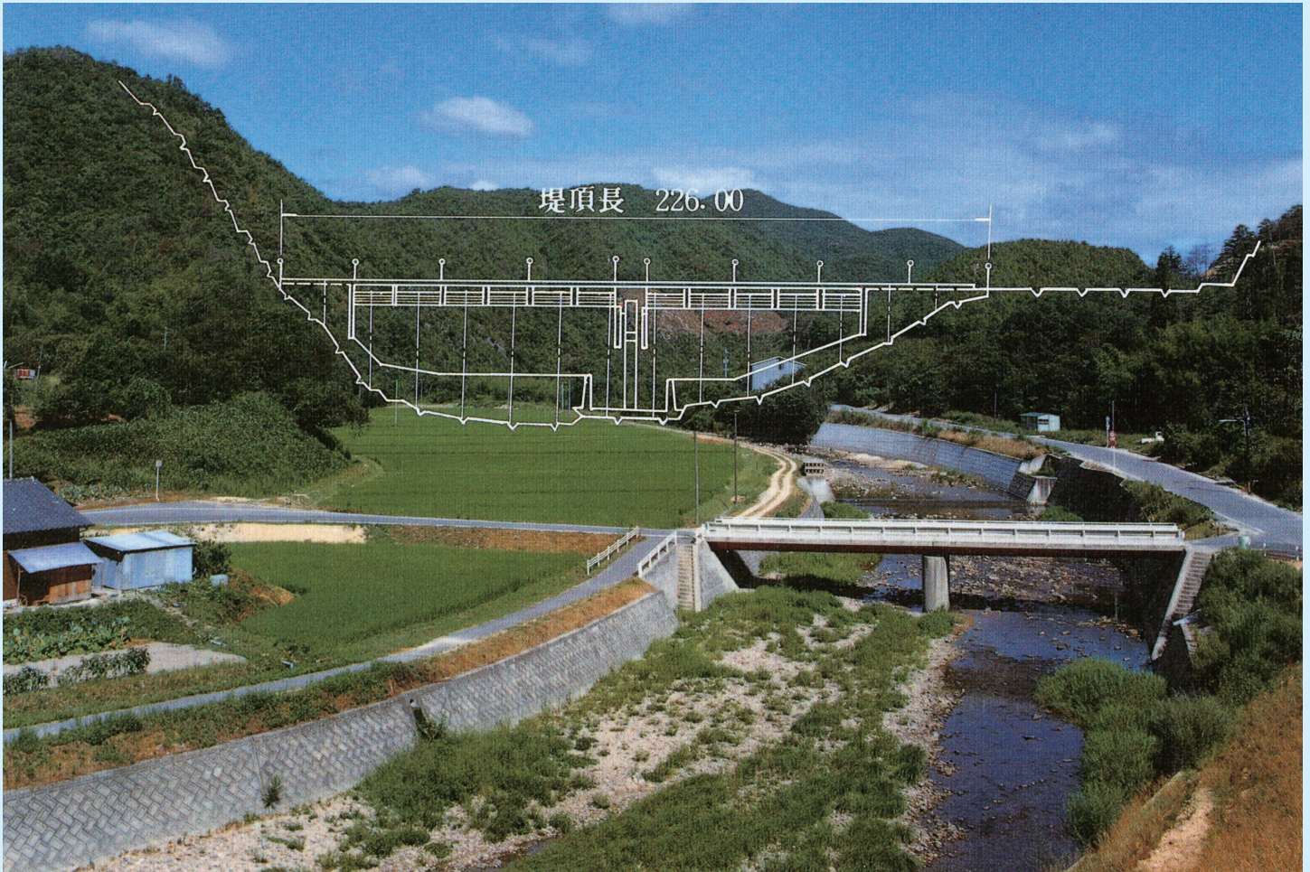
備前市 八塔寺川ダム地点を下流から望む〔完成予想図〕 昭和58年(1983)
